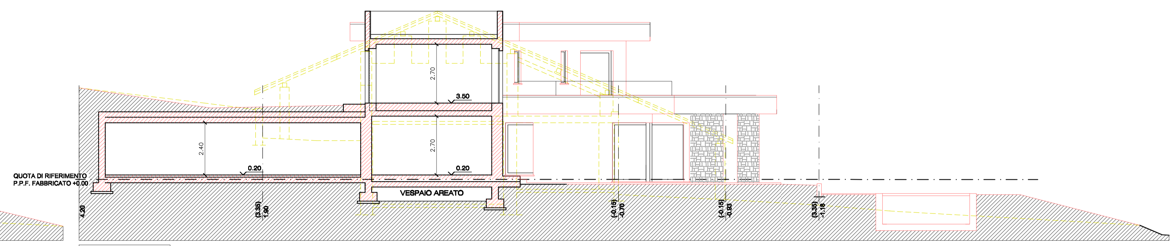
SEZIONE B-B
