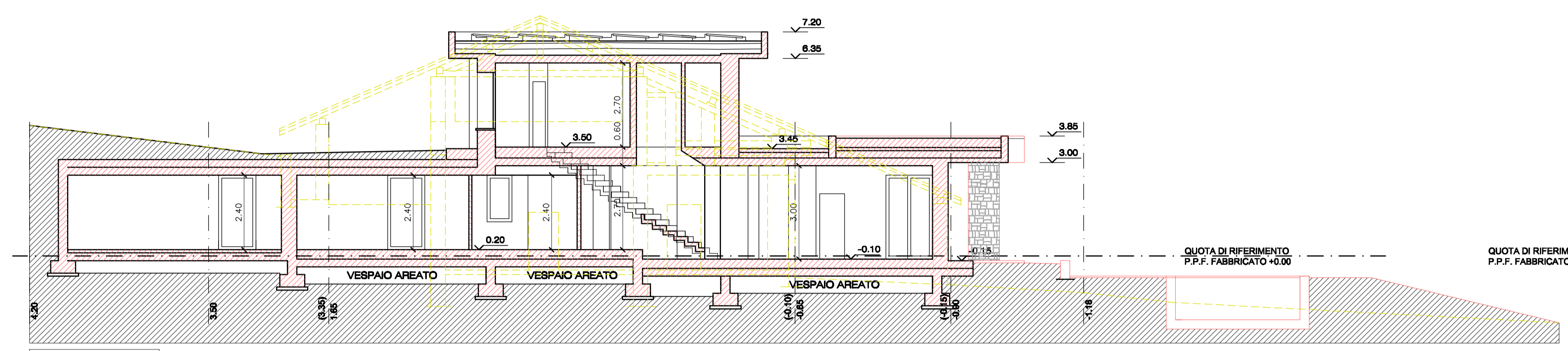
SEZIONE A-A
