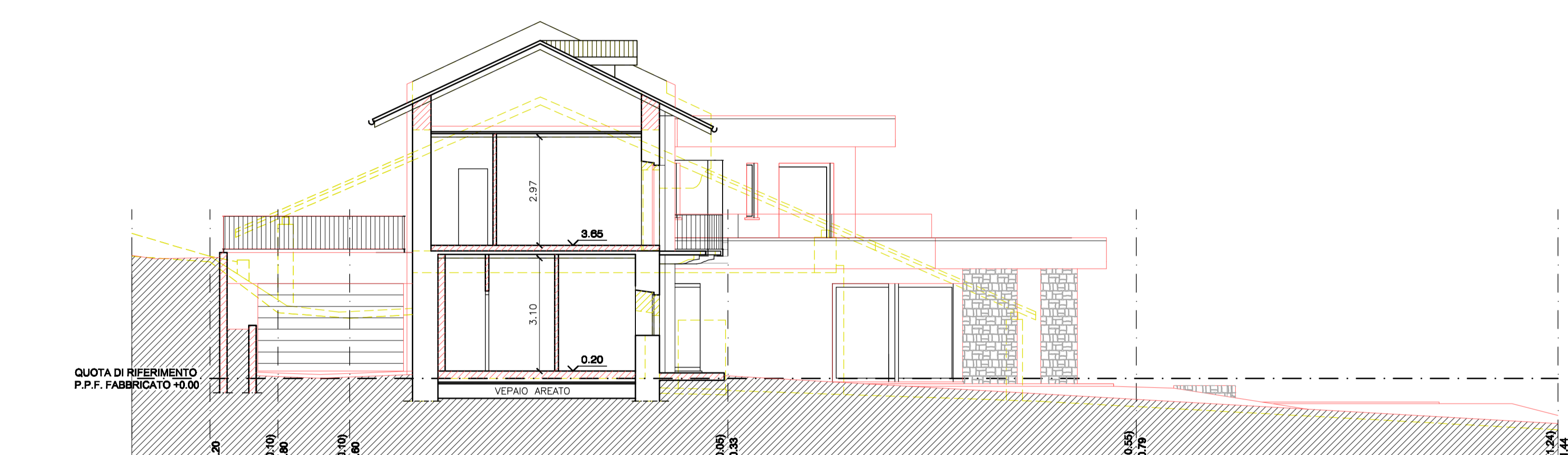
SEZIONE D-D
