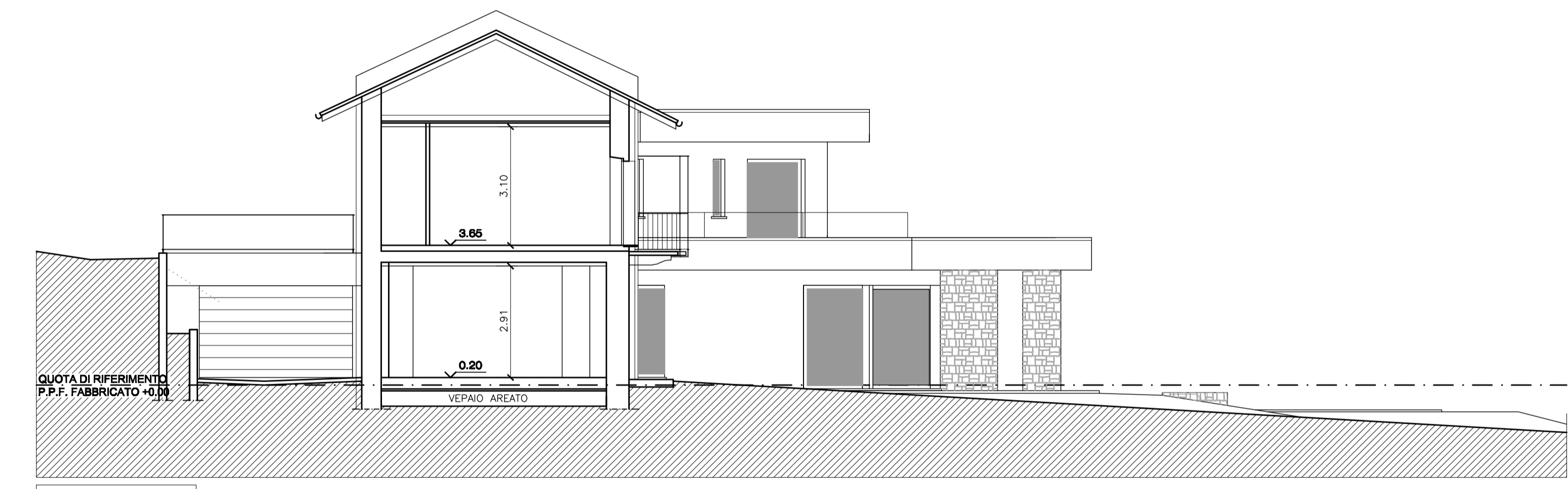
SEZIONE C-C
