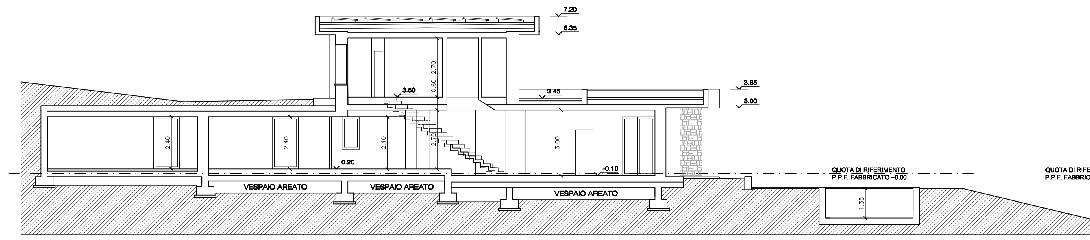
SEZIONE A-A
