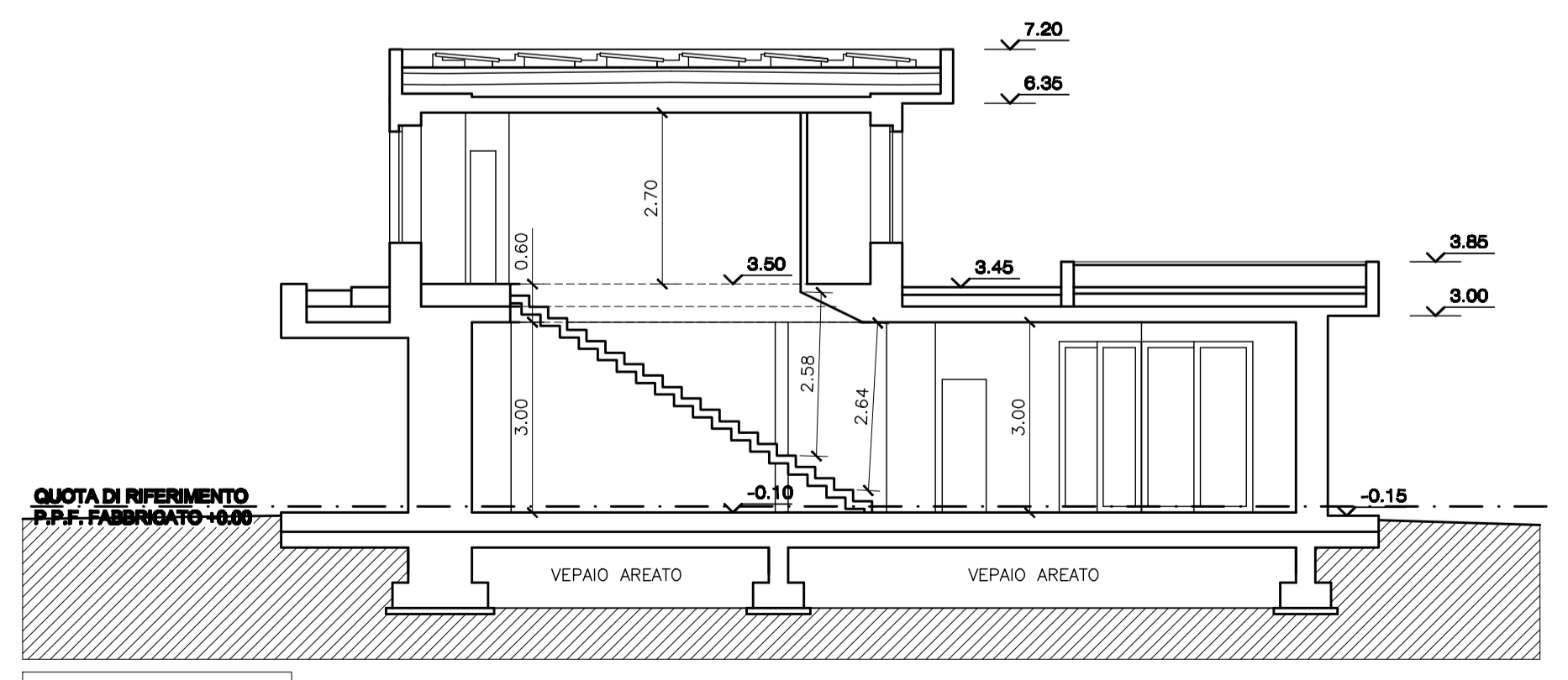
SEZIONE A1
