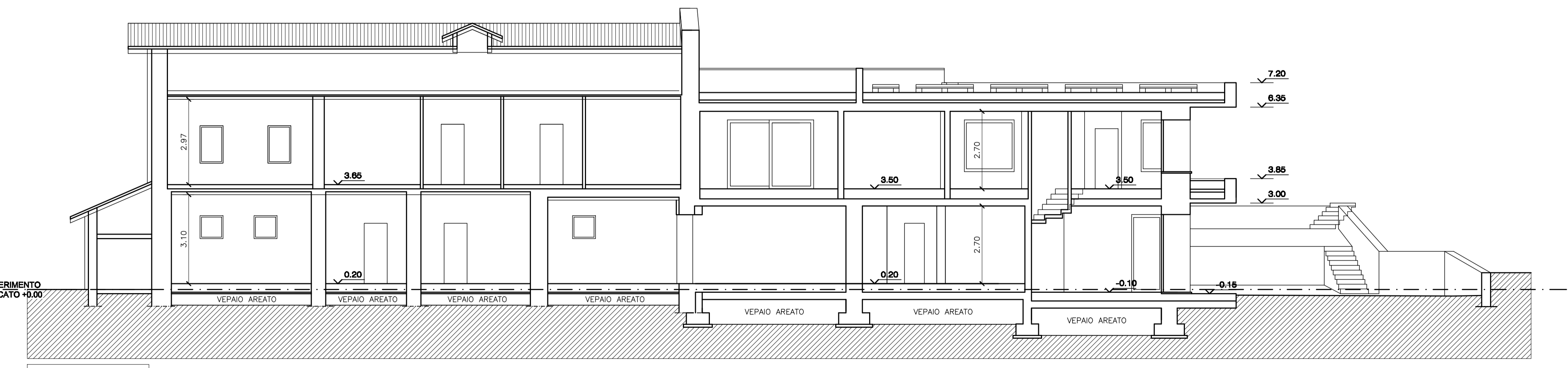
SEZIONE E-E
